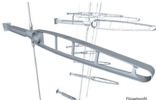
Flügelprofil
